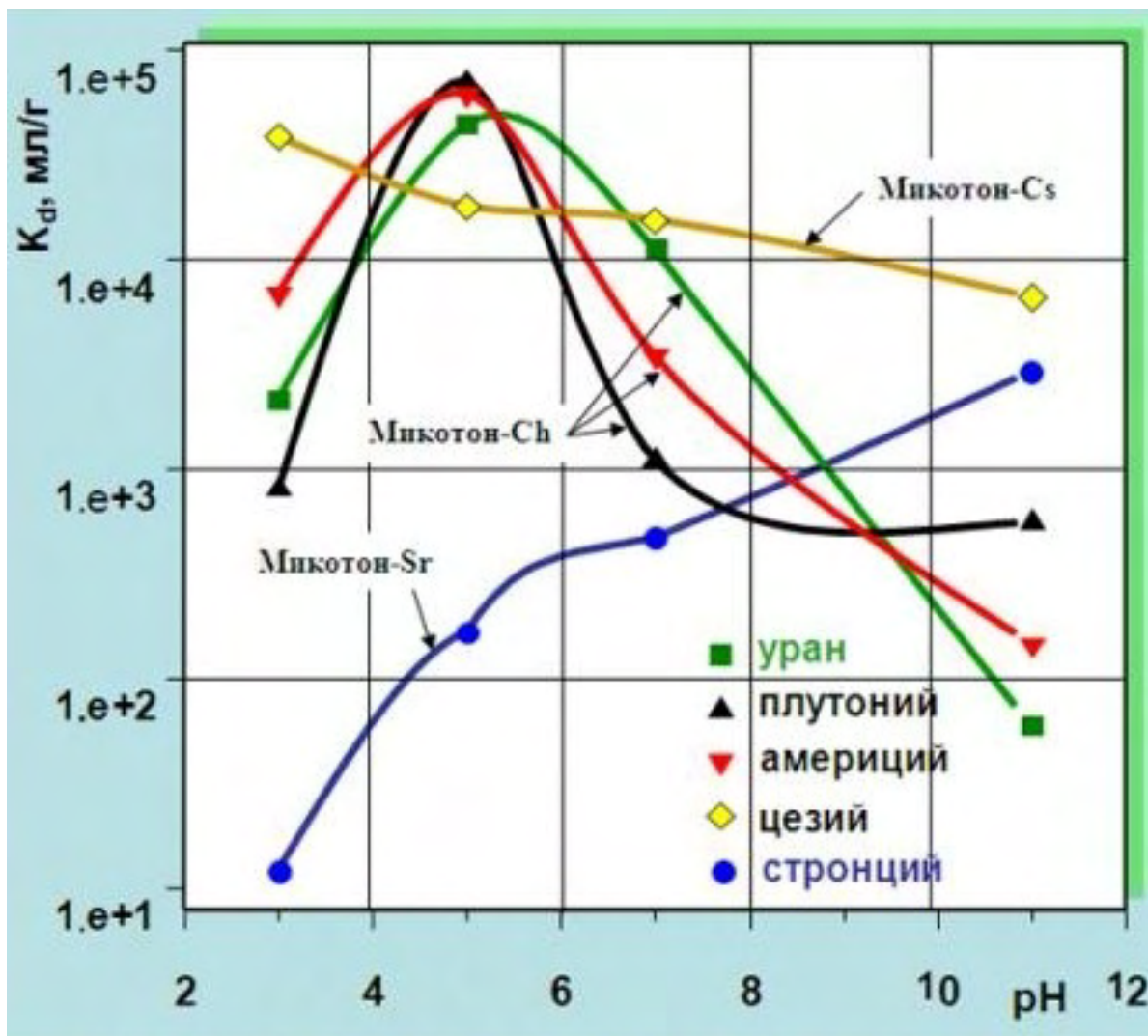
Рис. 20. Влияние pH раствора на сорбцию радионуклидов различными сорбентами Микотон
